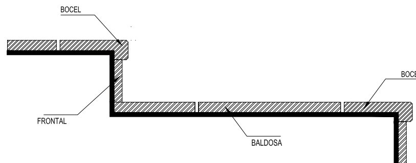
DETALLE CONSTRUCTIVO
