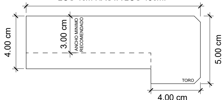
VISTA PERFIL
